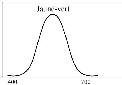
Sensibilité de l'oeil
