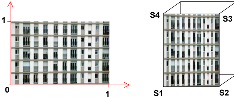
Image dans l'espace de texture et plaquage de cette image sur une face
