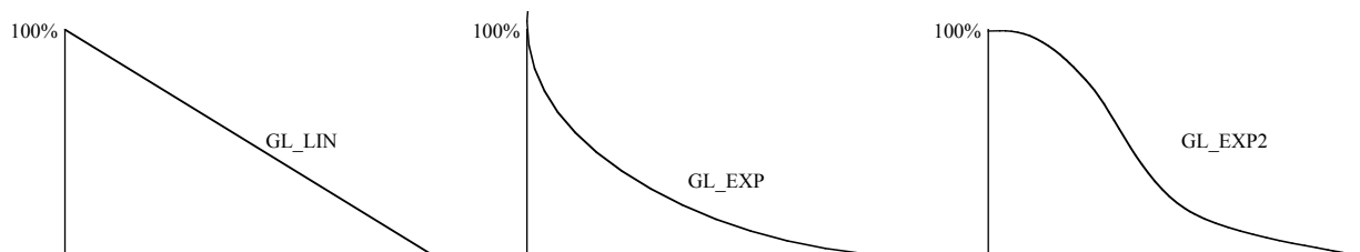
Pourcentage de la couleur d'origine d'après la distance au point de vue.
