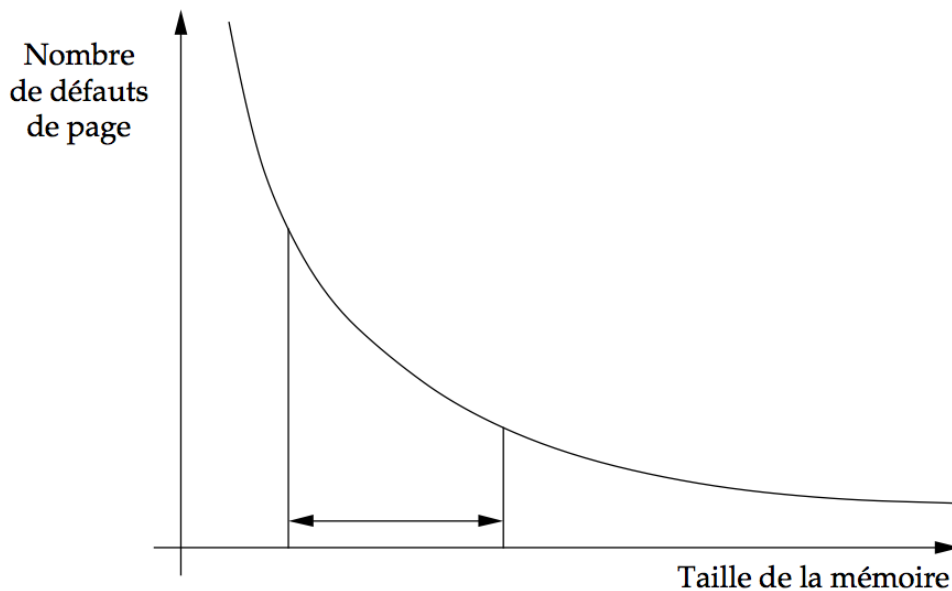
FIGURE 29: Nombre total de défauts de page en mémoire restreinte.
