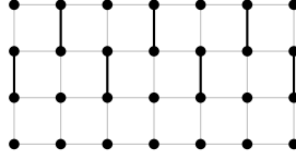
Figure 4: Matching M in G_{7,4} for Lemma 12.
